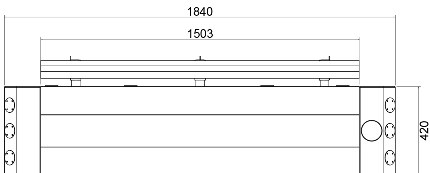
VISTA DALL'ALTO
