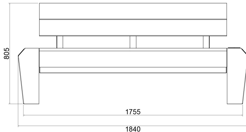
VISTA FRONTALE
