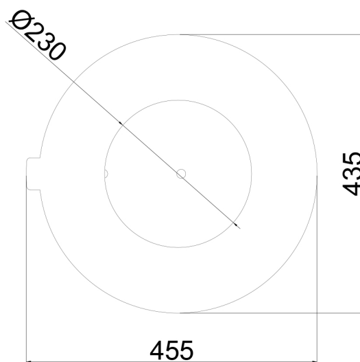
VISTA DALL'ALTO
