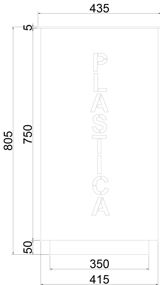
VISTA FRONTALE
