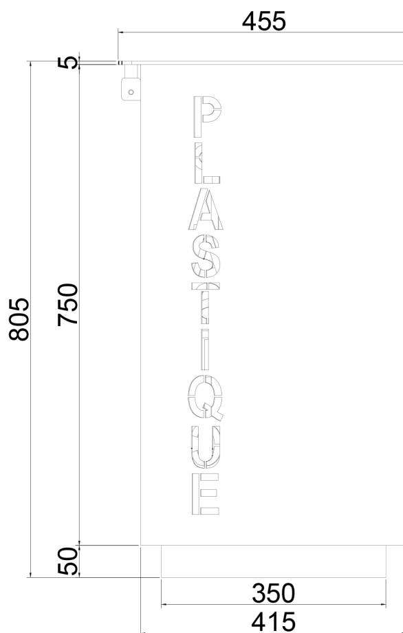
VISTA LATERALE
