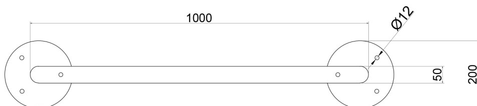
VISTA DALL'ALTO
