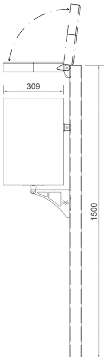
VISTA LATERALE
