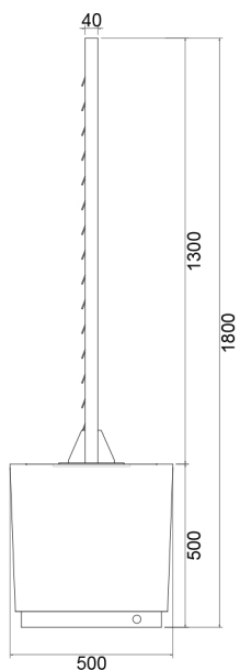
VISTA LATERALE
