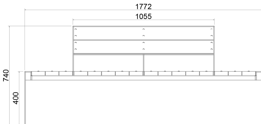
VISTA FRONTALE
