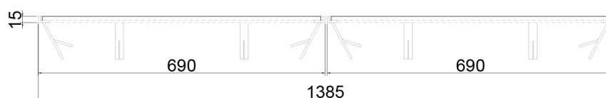
VISTA LATERALE
