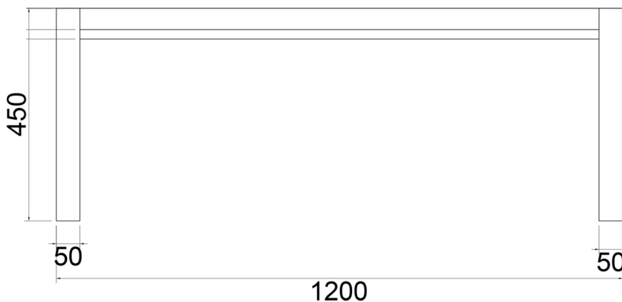
VISTA FRONTALE
