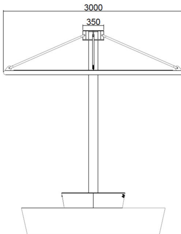
VISTA FRONTALE
