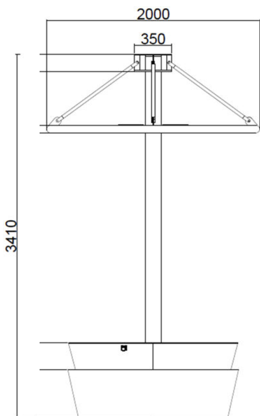
VISTA LATERALE
