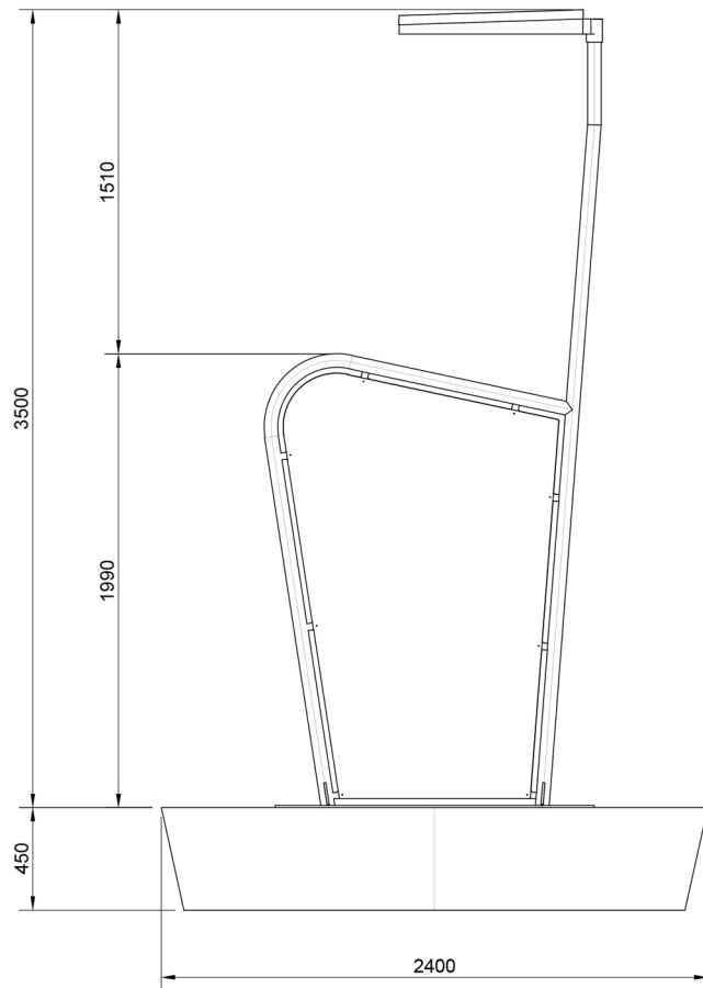
VISTA FRONTALE
