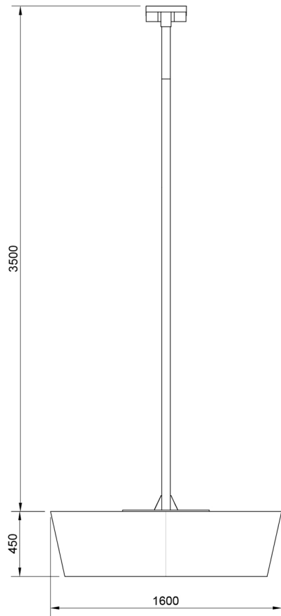
VISTA LATERALE
