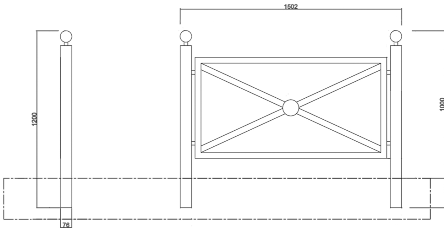
VISTA FRONTALE
