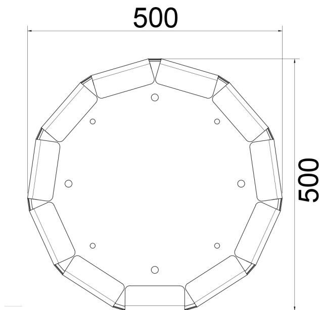
VISTA DALL'ALTO
