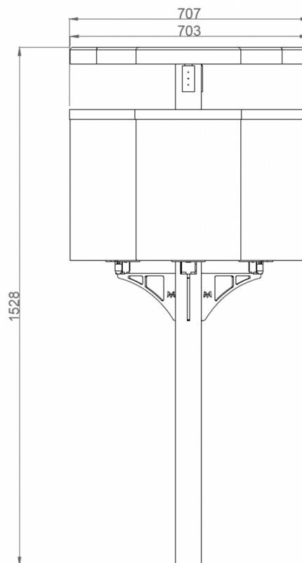
VISTA LATERALE
