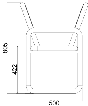
VISTA LATERALE
