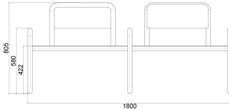
VISTA FRONTALE
