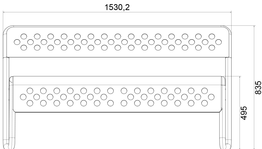
VISTA FRONTALE
