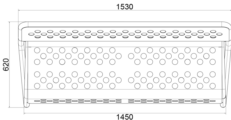
VISTA DALL'ALTO
