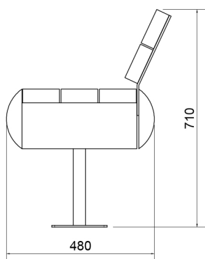
VISTA LATERALE
