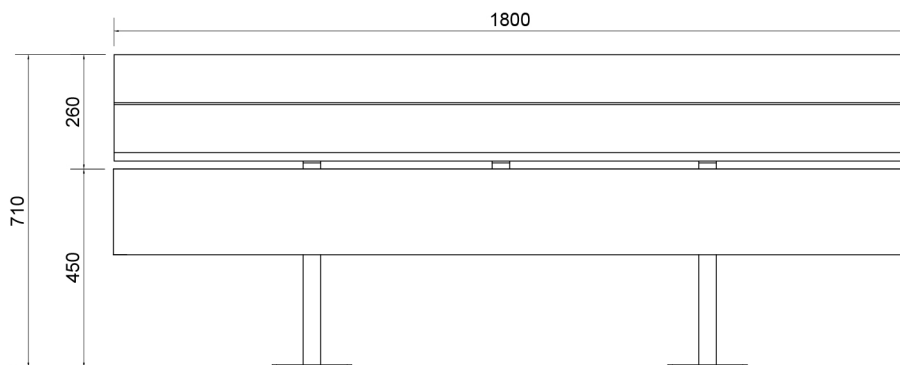
VISTA FRONTALE
