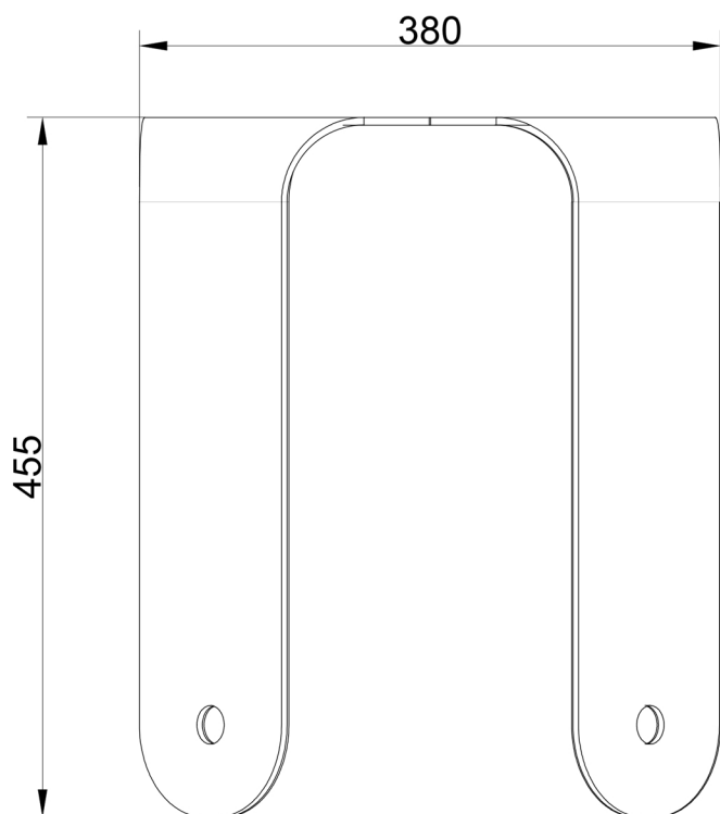
VISTA LATERALE
