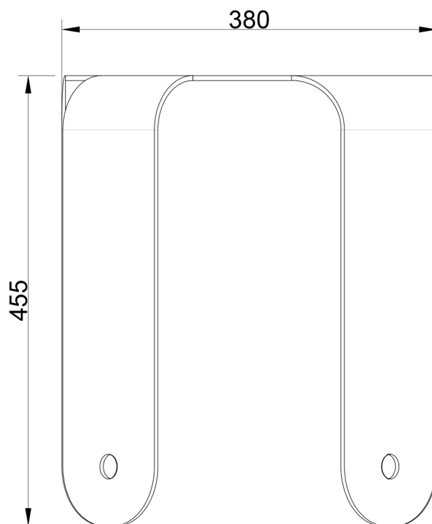
VISTA FRONTALE
