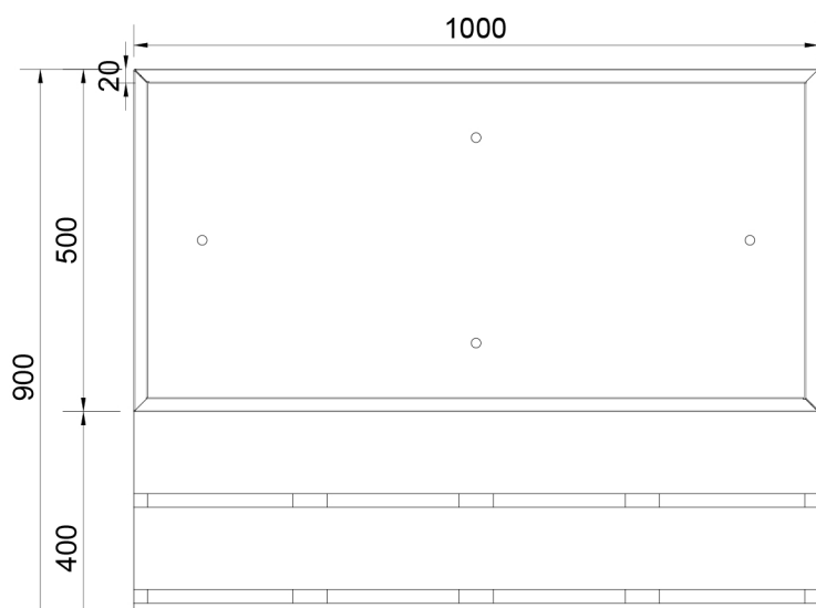
VISTA DALL'ALTO
