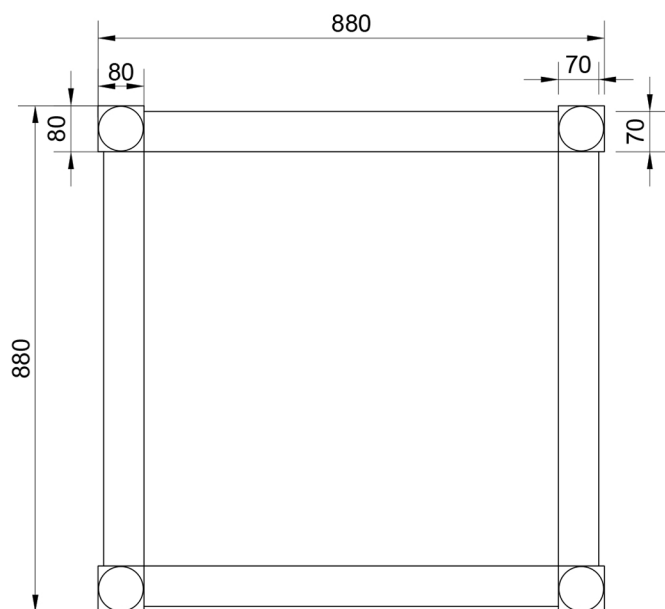
VISTA DALL'ALTO
